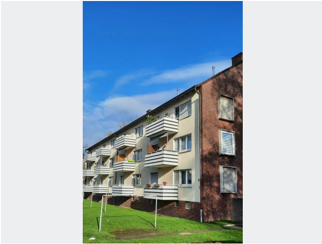
Außenansicht Balkone
